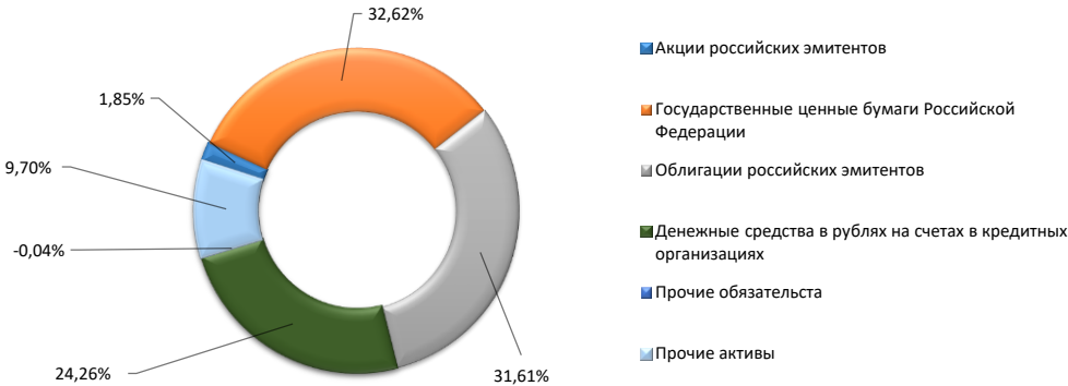
Структура средств пенсионных резервов фонда на 28.02.2025
